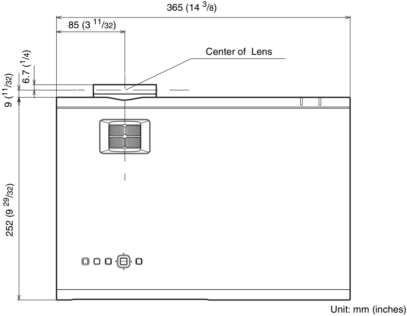
Top (VPL-EW295)
