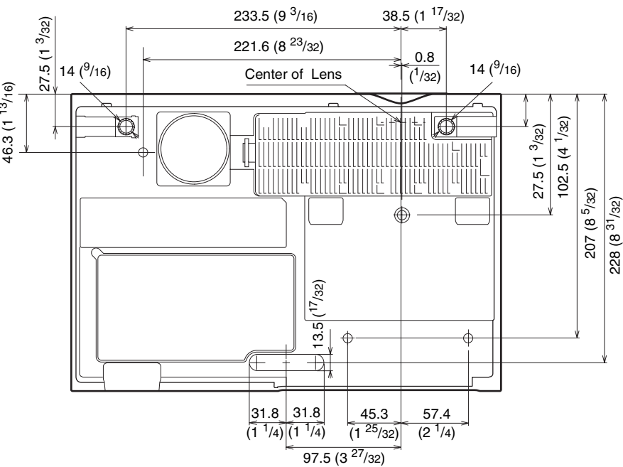
Bottom (VPL-EW235/EX250/EX235/EX230)
