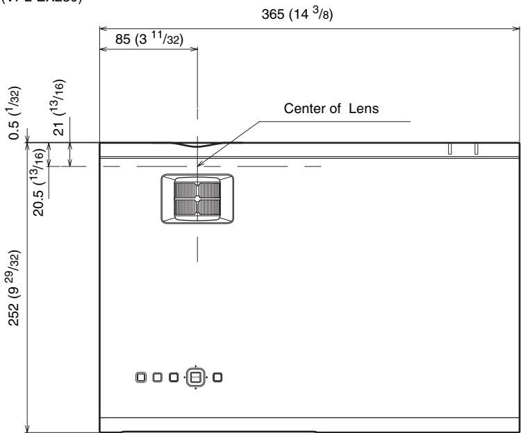
Top (VPL-EX230)
