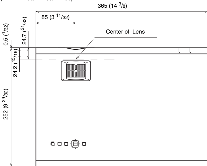
Top (VPL-EW235/EX250/EX235)
