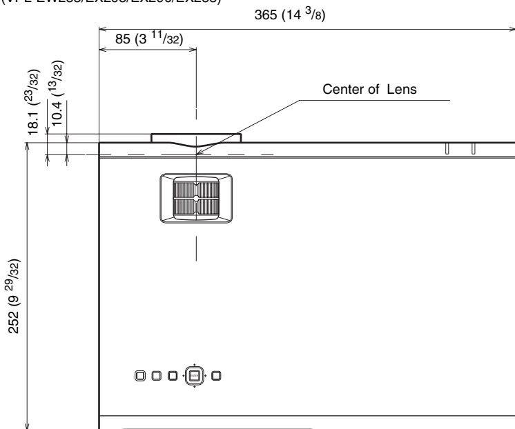
Top (VPL-EW255/EX295/EX290/EX255)
